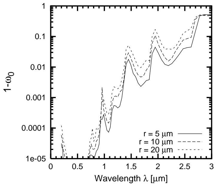
(d) Single Scatter Co-Albedo - Cloud Droplets
