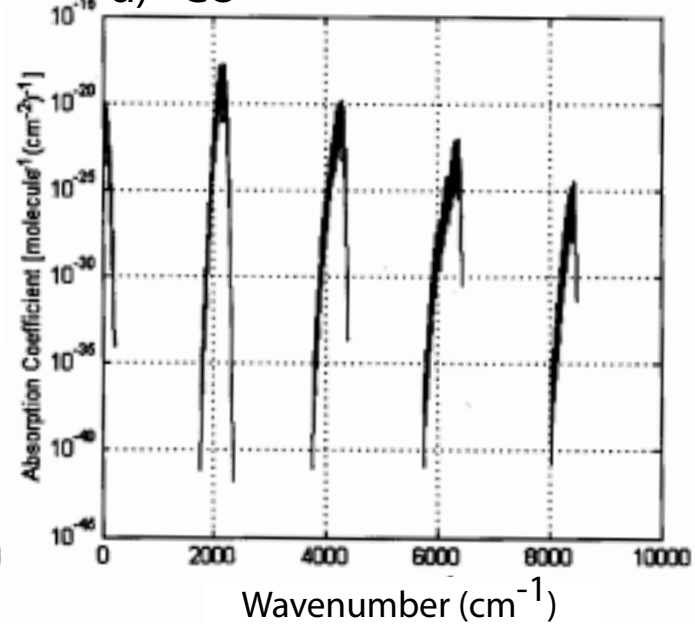
d) CO
