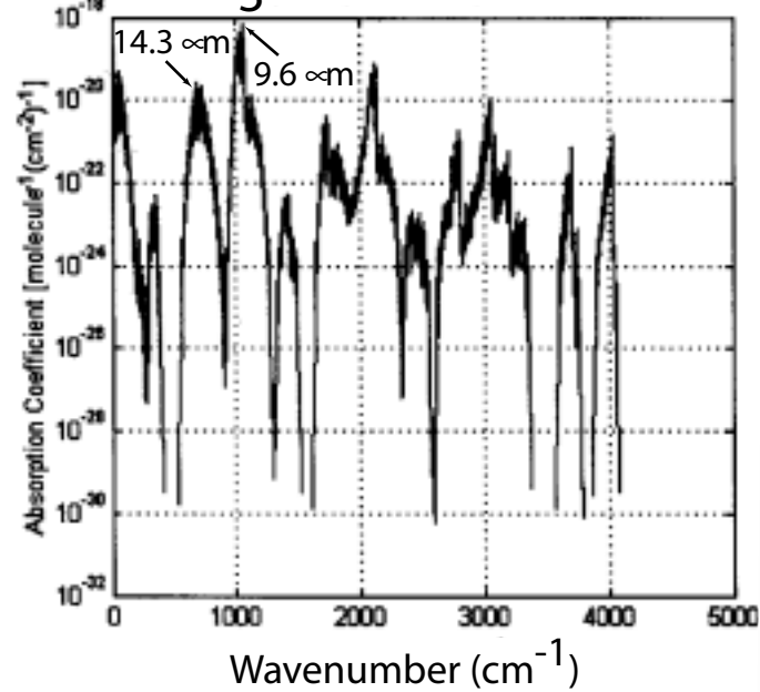
c) O 3
