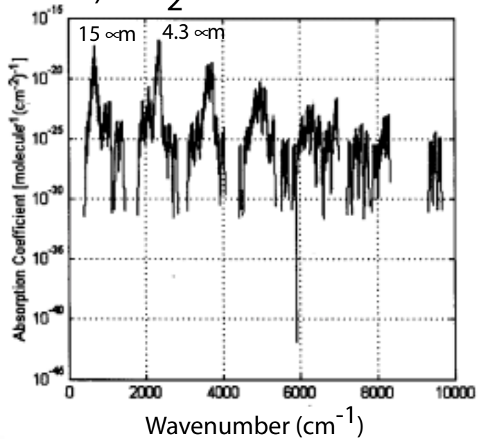
b) CO 2
